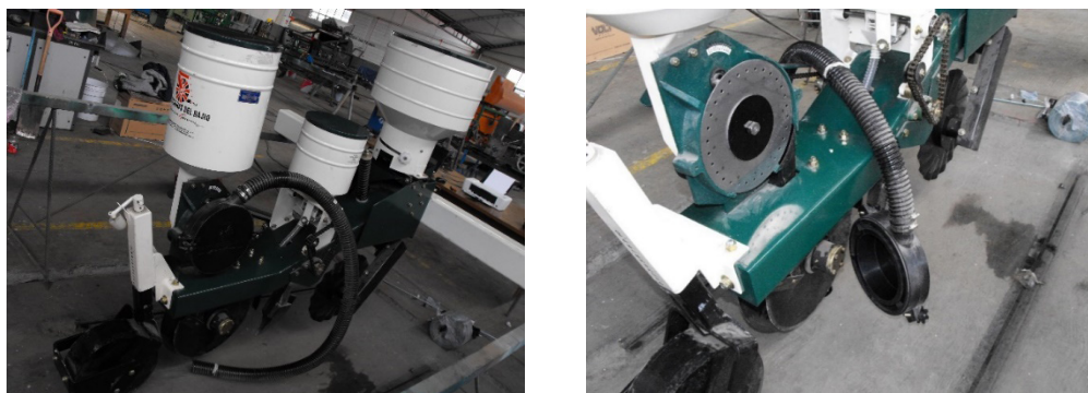
A) Cuerpo sembradora-fertilizadora. B) Vista del sistema neumático.
