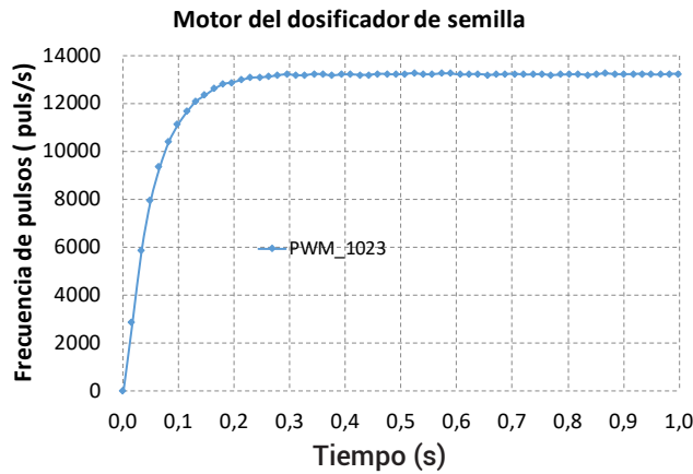
A) Respuesta del sistema a una entrada escalón.
