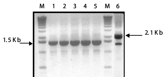
Figura 2. Ensayo por PCR en plantas transgénicas de A. thaliana . Se muestra la amplificación de una región del T-ADN de las construcciones pBADH-GUS-NOS (carriles 1-5) y pBI121 (carril 6). Para amplificar la región de 1.5 Kb del promotor del gen ahybadh4 (carriles 1-5) se utilizaron los oligonucleótidos M13 reverso y ahybadh4 . Para obtener el fragmento de 2.1 kb del gen reportero GUS (carril 6) se utilizaron los oligonucleótidos 35S y M13 universal. M: marcadores de peso molecular (1 Kb ladder, Gibco BRL).
