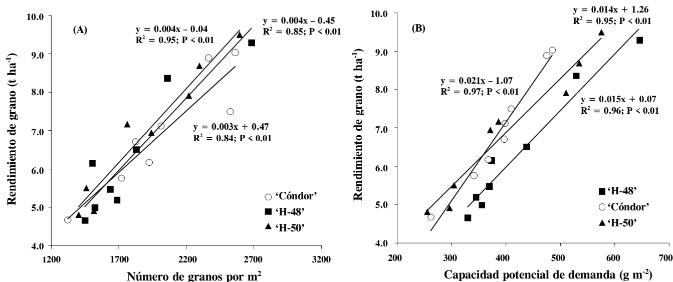
Figura 2. Relación entre el rendimiento de grano con el número de granos por m 2 (A) y la capacidad potencial de demanda (B). Los puntos representan a la respuesta de cada híbrido a través de los ocho ambientes de evaluación (n = 3).
